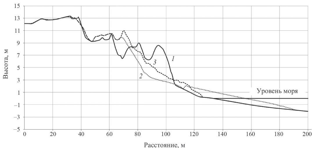
Рис. 11. Переформирование профиля 3 различными штормами при разных уровнях (увеличенный масштаб приустьевой зоны).
