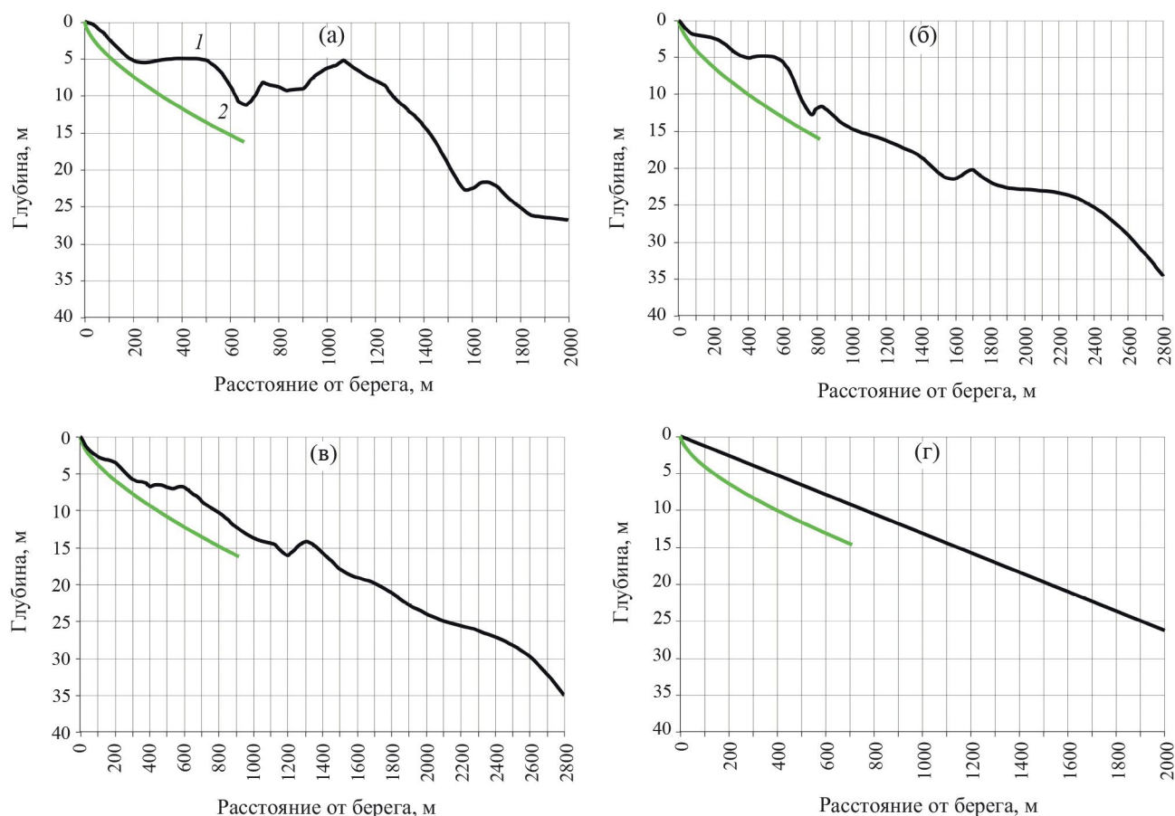
Рис. 7. Результаты моделирования профилей динамического равновесия для Курильского залива.
