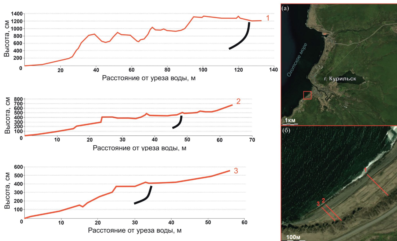
Рис. 4. Профили берега (урез моря слева) и расположение погребенных уступов (черные линии — предполагаемое положение в почвенно-пирокластическом чехле).
