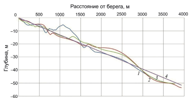
Рис. 6. Профили подводного берегового склона Курильского залива и линейный тренд (средний профиль).
