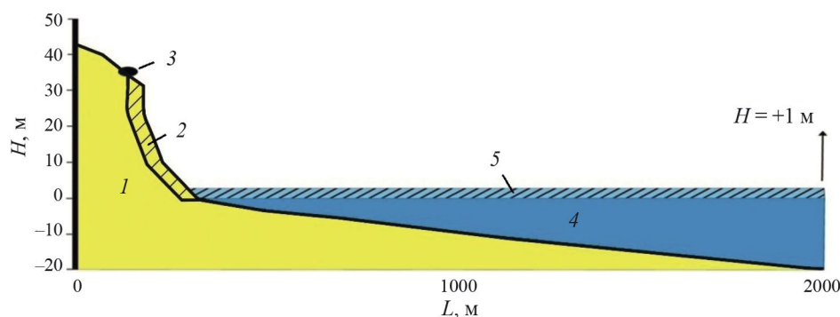
Рис. 8. Возможное переформирование берега Курильского залива после подъема относительного уровня моря на 1 м в результате гидродинамических и геодинамических факторов.
