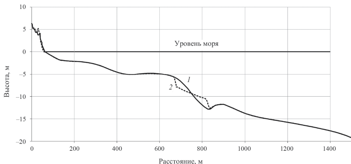
Рис. 10. Переформирование профиля 2 штормом 2%-ной повторяемости (172 ч/год, H = 5 м). 1 – исходный профиль; 2 – шторм 2%-повторяемости, H = 5 м.
