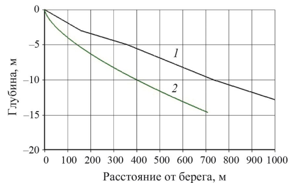
Рис. 5. Результаты моделирования профиля динамического равновесия для Курильского залива. 1 – исходный подводный береговой склон; 2 – теоретический профиль динамического равновесия по модели Дина.
